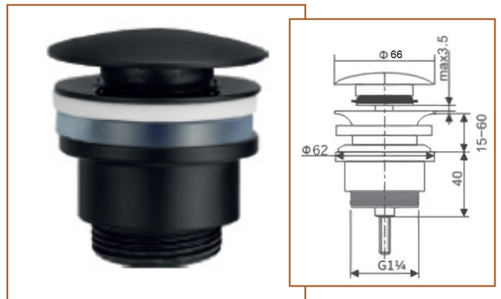
VALVULA CLIC CLAC NEGRA VCC008 14,50 €
