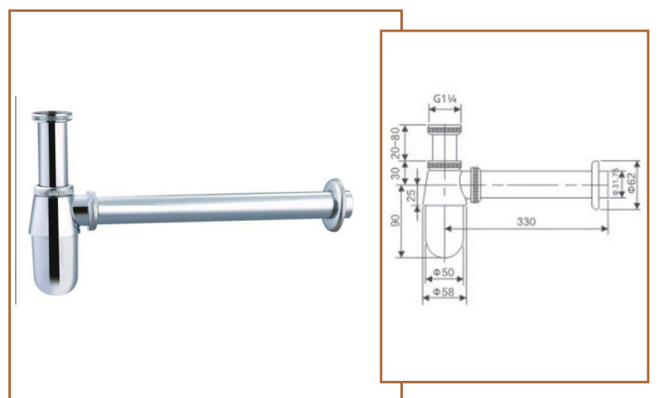
SIFÓN CROMADO VISTO REDONDO SCL001 10,50 € » ACERO INOX 304 Y ZAMAK
